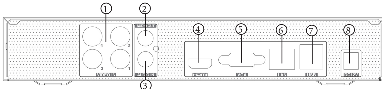
Задняя панель CTV-HD924 HP Lite
