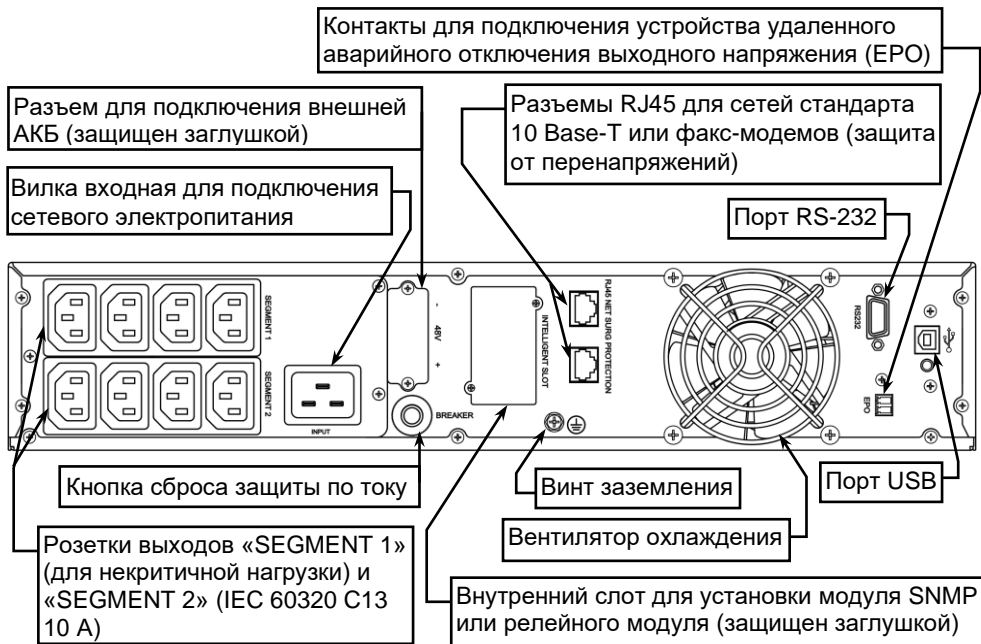
Рисунок 2 – Общий вид задней панели изделия
