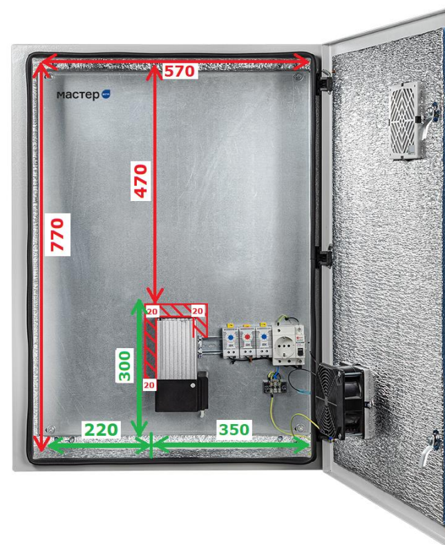
Нагреватель на 250Вт
