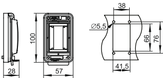
Рисунок 1. Основные размеры крышек.
