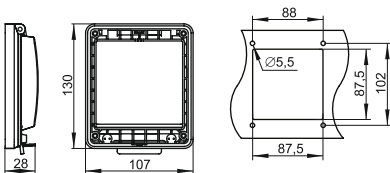
Рисунок 1. Основные размеры крышек (продолжение).
