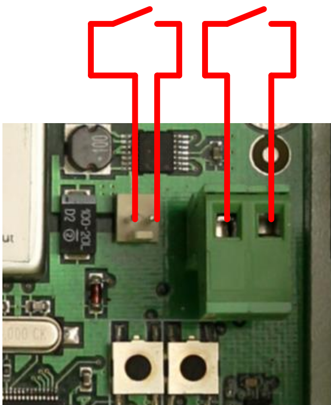
Рис. 2.6. Сухие контакты
