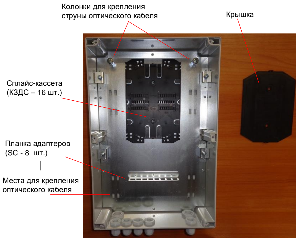
Рис. 2.4. Оптический кросс
