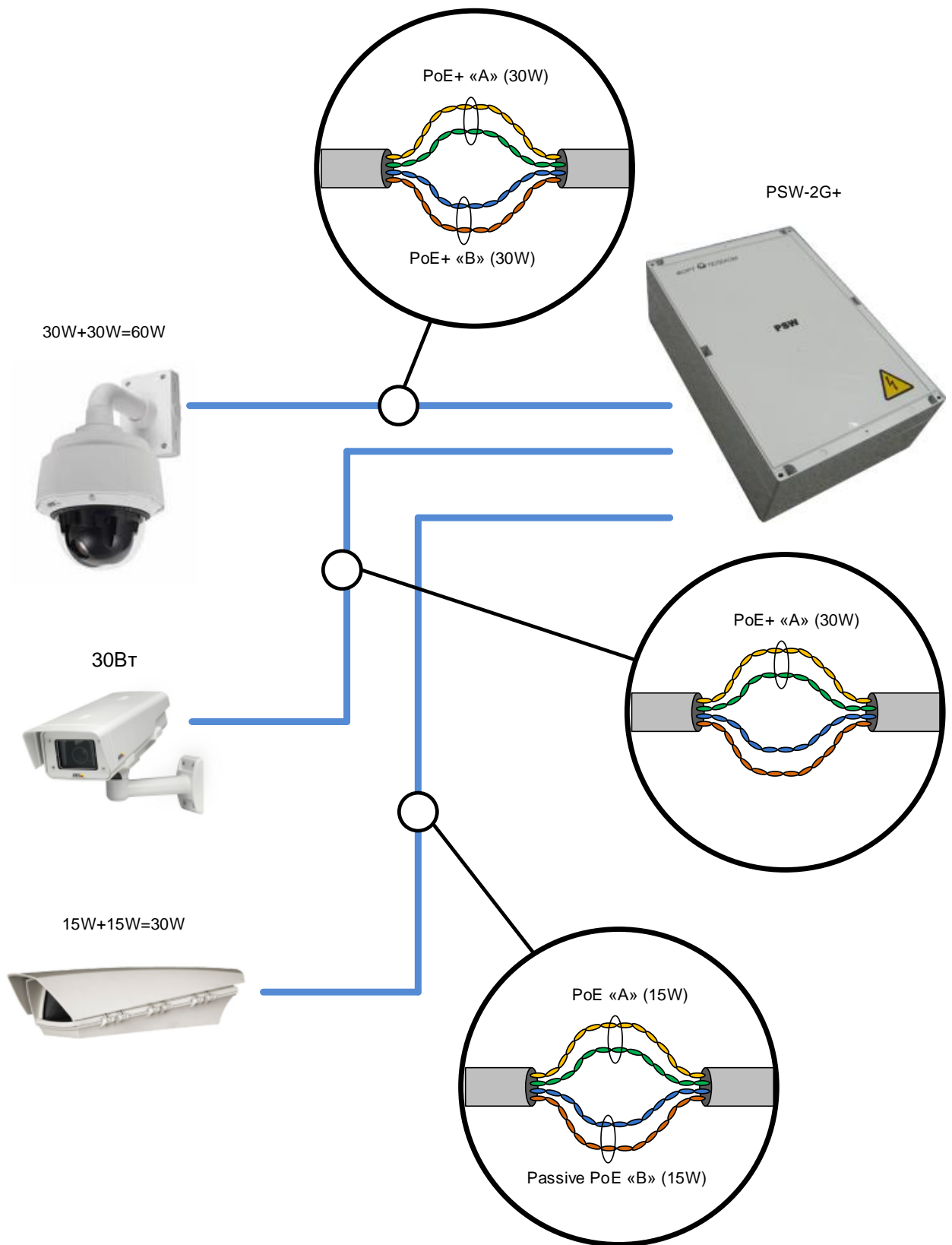
Рис. 2.3. Схема питания по PoE для разных случаев
