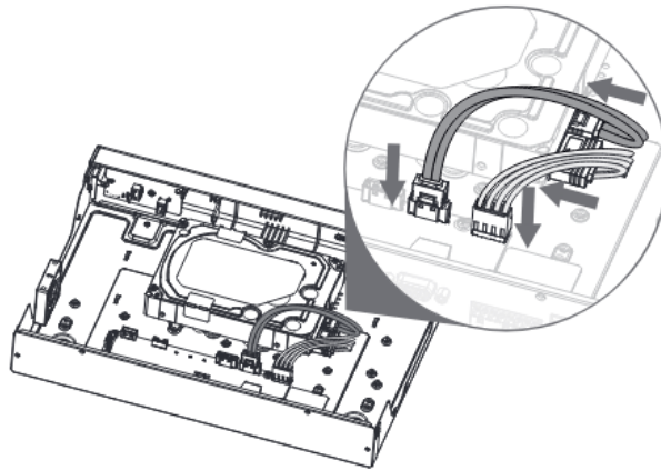
Рисунок 3.7 – Установка жесткого диска
