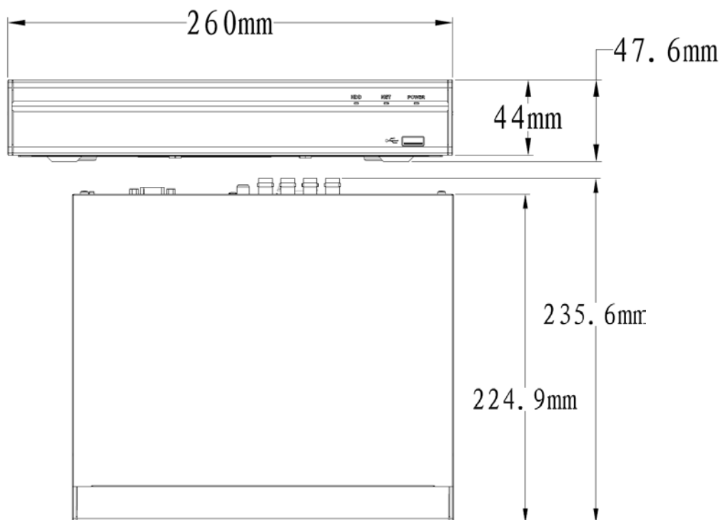
Рисунок 3.9 – Габаритные размеры видеореєстратора
