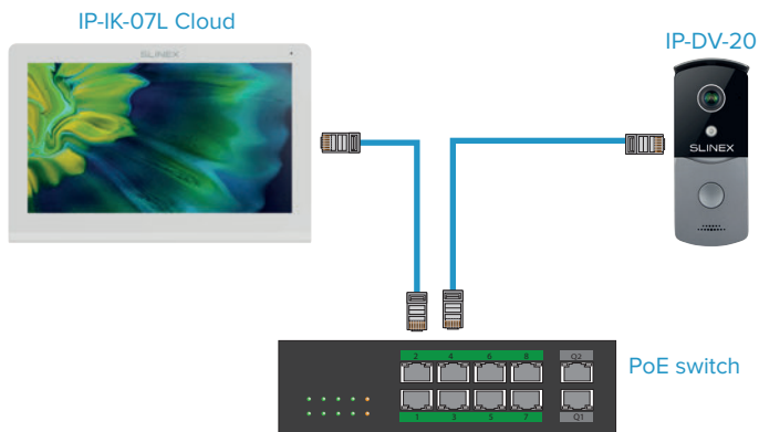
Схема 1. Топология подключения IP системы видеодомофони.
