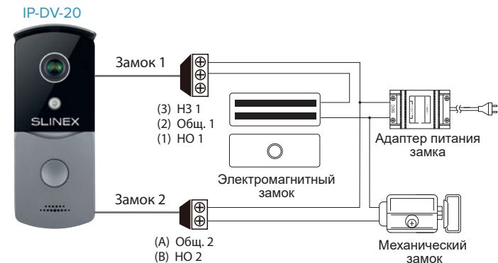
Схема 3. Подключение замков с питанием от внешнего адаптера.
