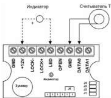
Пример подключения TM
